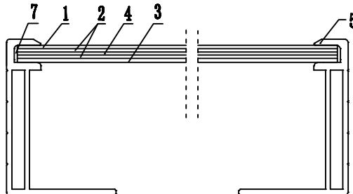
A-A 处放大图 10:1
